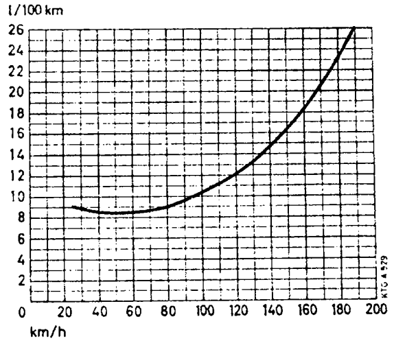
Kraftstoffverbrauch, Belastung 2 Personen
