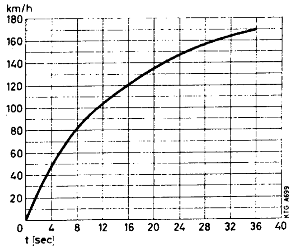
Beschleunigung mit Durchschalten * Belastung 2 Personen
