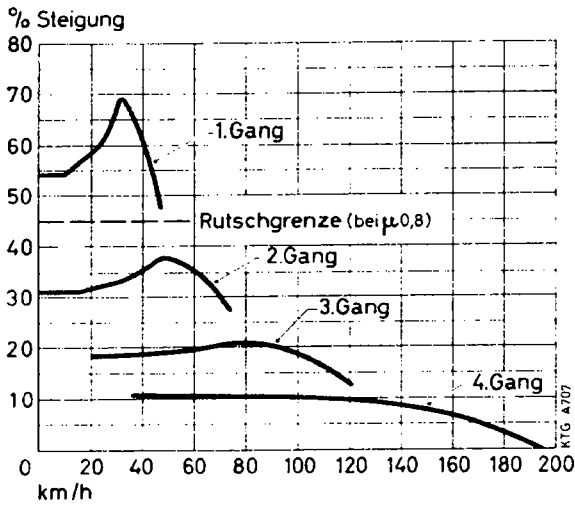
Steigfähigkeit, Belastung 2 Personen * (Coupé)
