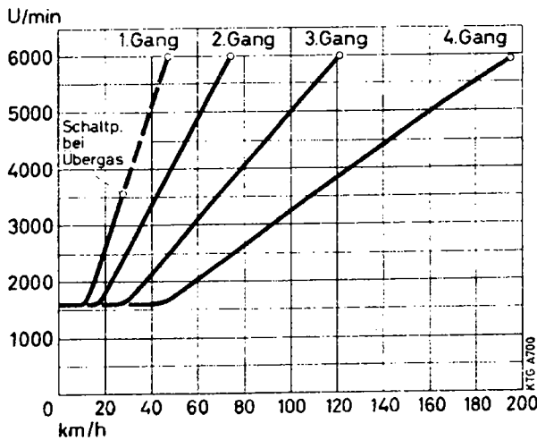
Ganggeschwindigkeit und Motordrehzahl *
