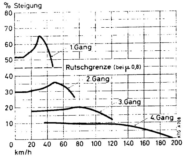
Steigfähigkeit, Belastung 2 Personen * (Cabriolet)
