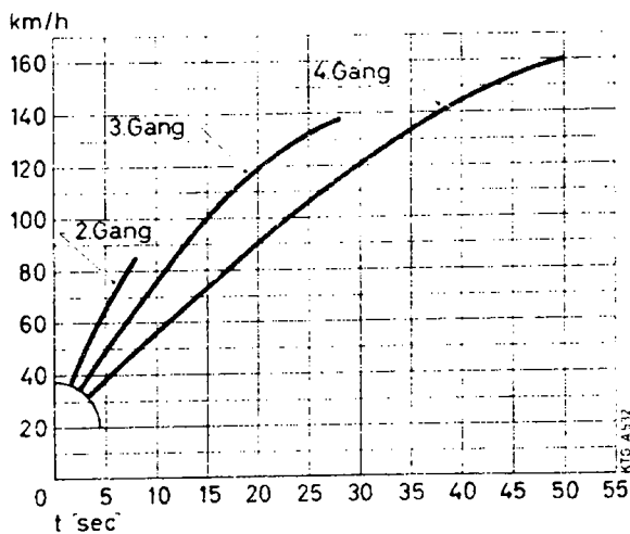
Beschleunigung in den einzelnen Gängen Belastung 2 Personen
