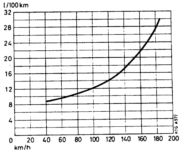
Kraftstoffverbrauch, Belastung 2 Personen *
