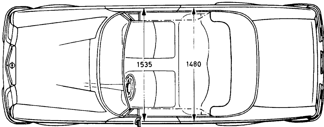
Innenmaße unbelastet
