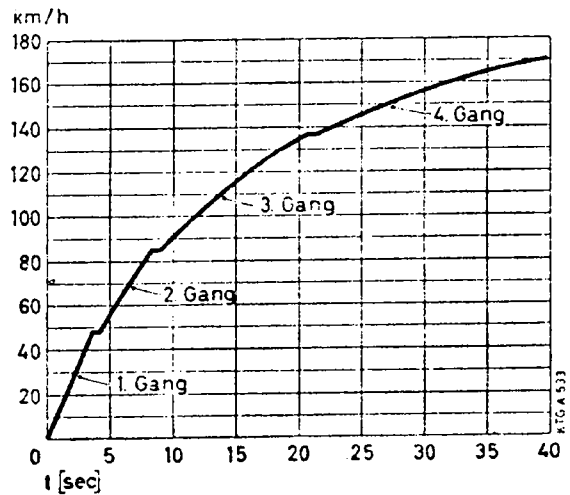
Beschleunigung mit Durchschalten Belastung 2 Personen
