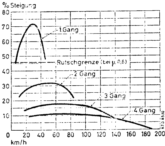
Steigfähigkeit, Belastung 2 Personen
