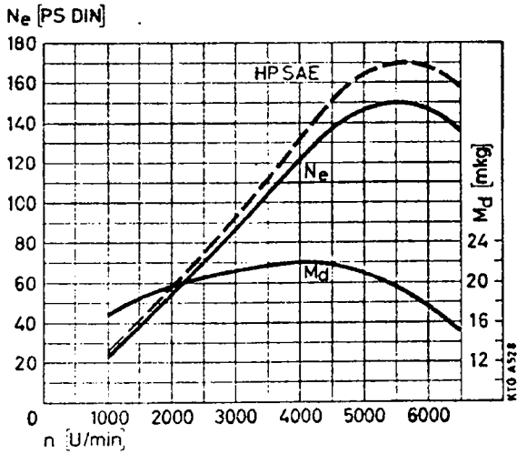
Leistung, Drehmoment und effektiver Druck
